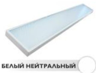
Светодиодный светильник HTF-001 1190x150x30 с аварийным блоком питания 32W 220V IP40 OSR (NW)
